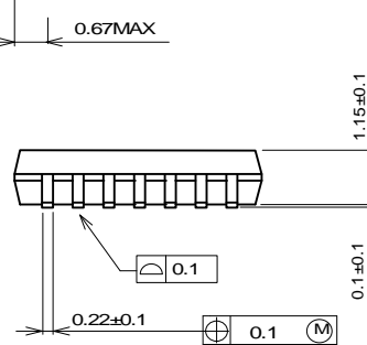
SSOP14 Package
