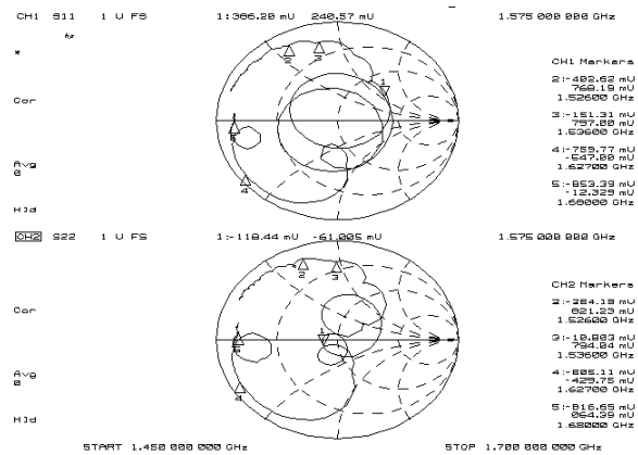
Zin, Zout
